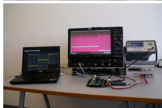
Abbildung 8: EM-Sonde zum Messen der elektromagnetischen Abstrahlung auf einem geöffneten Chip (Mitte), Messplatz zur Poweranalyse eines Mikrocontrollers und FPGA-Platine zu dessen Steuerung (oben und unten) im Testlabor des Fraunhofer SIT-München
